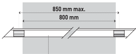
Section profilé STARLINE (800 mm) spécialement usiné pour gaine technique (autres dimensions sur demande)
